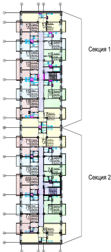
План 2 этажа
